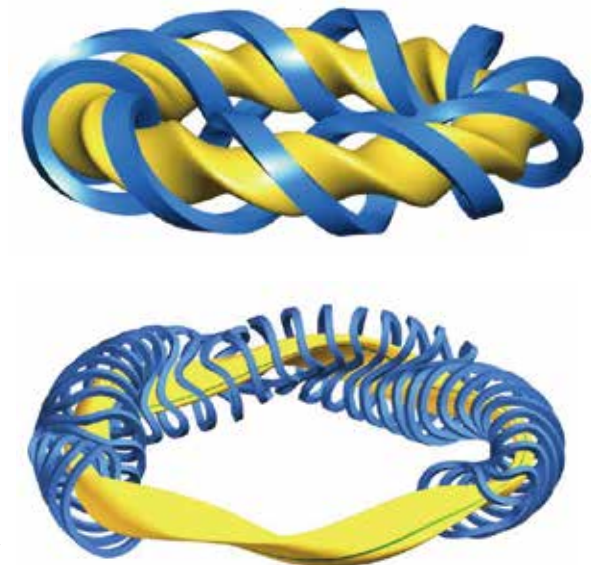
LHD（上）とW7-X（下）の電磁石（青）とプラズマ（黄）の形 （W7-Xの画像はマックス・プランク・プラズマ物理研究所より提供）
